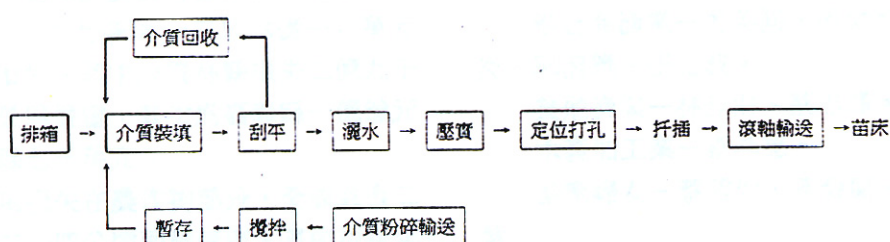
圖 1 菊花穴盤扦插育苗機械作業系統流程圖
