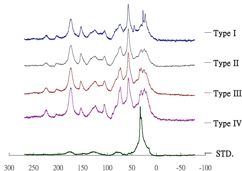
圖 1. 不同堆肥的腐植酸之 ^{13}\text{C} 固態核磁共振光譜
