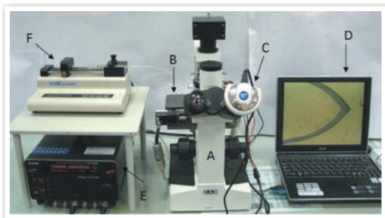
❶ 圖1. 實驗硬體設備 A.倒立式顯微鏡、B.移動平台、C.顯微影像電子目鏡、D.筆記型電腦、E.訊號產生器、F.微量注射幫浦及微量注射針筒。
