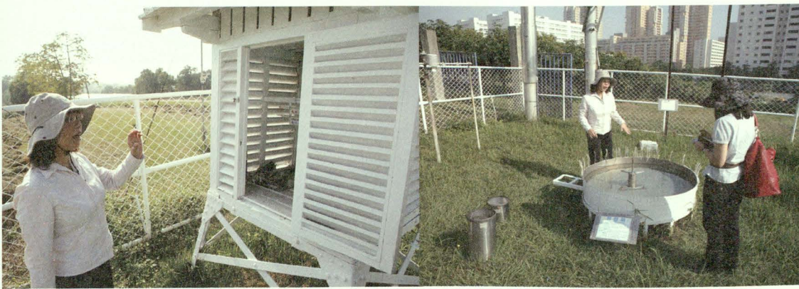
農業氣象觀測站
