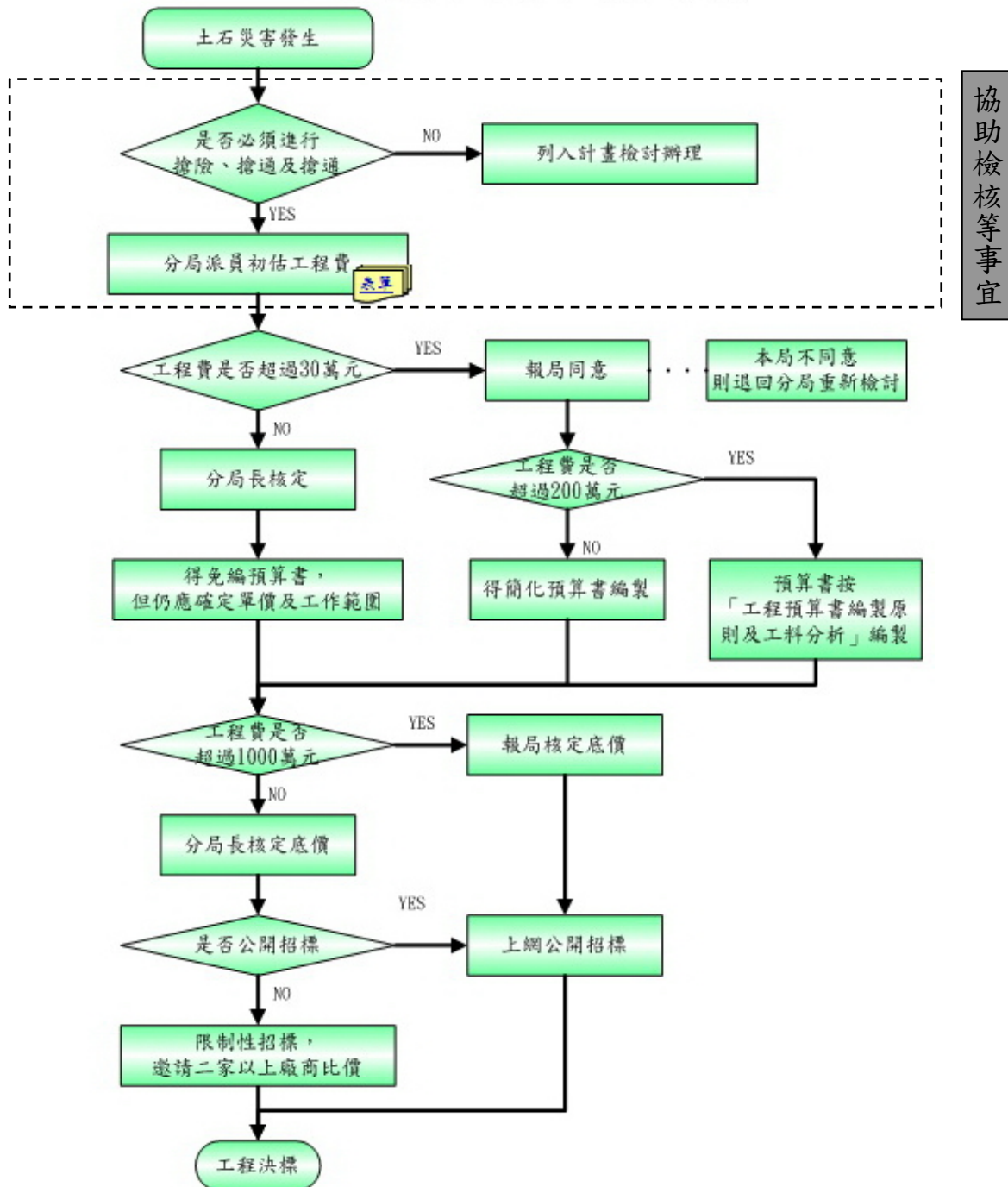
圖 7-2 防汛期間緊急處理委辦工程檢核流程圖
