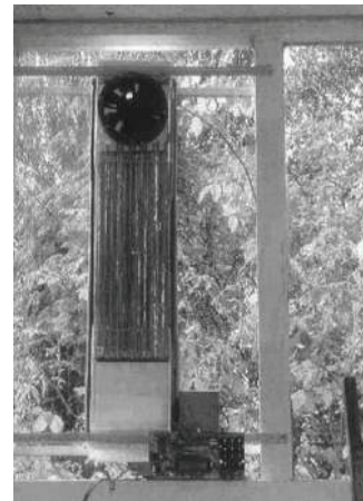
圖 4. 捲繞式空氣/空氣熱交換器之最先概念(上)與置於建築物正面之呼吸窗雛型(下)(Kristinsson, 2006a)
