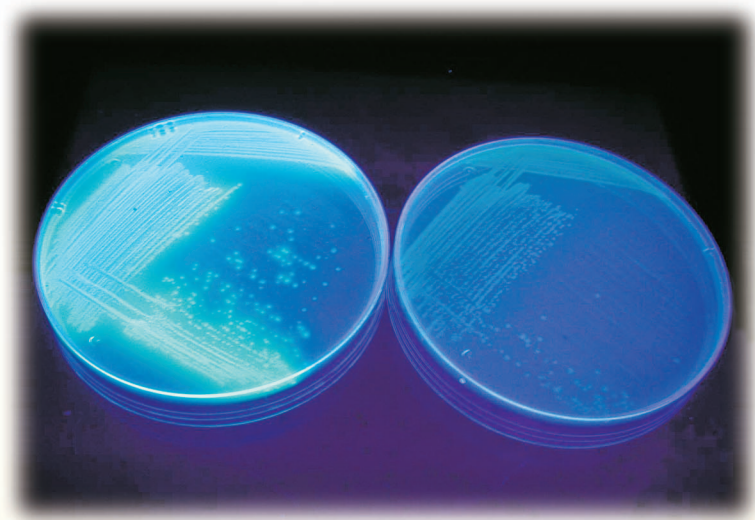
▲ 圖8. 以螢光假單胞菌( Pseudomonas fluorescens )來防治番茄青枯病(左方為螢光假單胞菌)。
