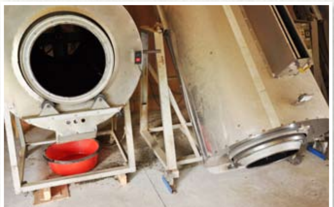
圖一、炒菁機後方，茶毛灰塵堆積
