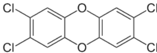
圖一、2,3,7,8-四氯雙苯環戴奧辛 (TCDD) 的結構式
