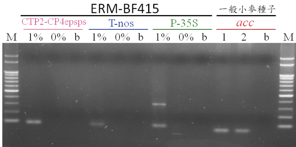
圖一、基因轉殖小麥(MON71800)定性檢測方法
