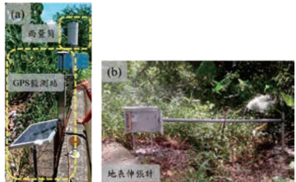
▲圖5、(a)GPS監測站及雨量筒，(b)地表伸張計。
