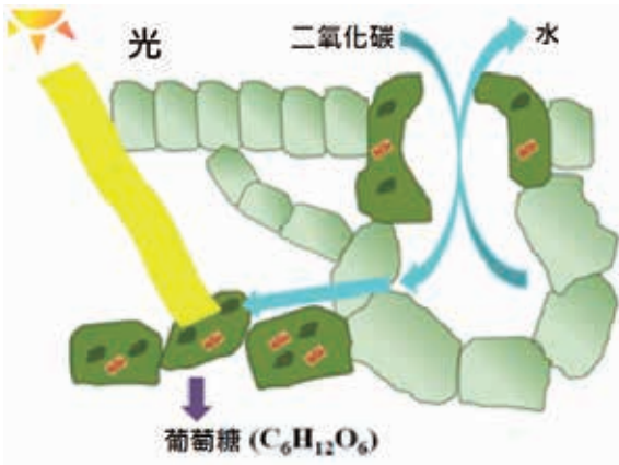
▲圖1、光合作用示意圖（修改自Nelson and Cox, 2009）。植物，通常會吸取大氣中的 CO_2 ，並藉由葉綠體將光的能量轉換，遂合成葡萄糖( C_6H_{12}O_6 )再以不同之酵素，進行生化反應，轉化成其他醣類，供給植物做結構或是非結構性碳水化合物，加以運用或儲存。此過程形成基礎的生物碳循環。
