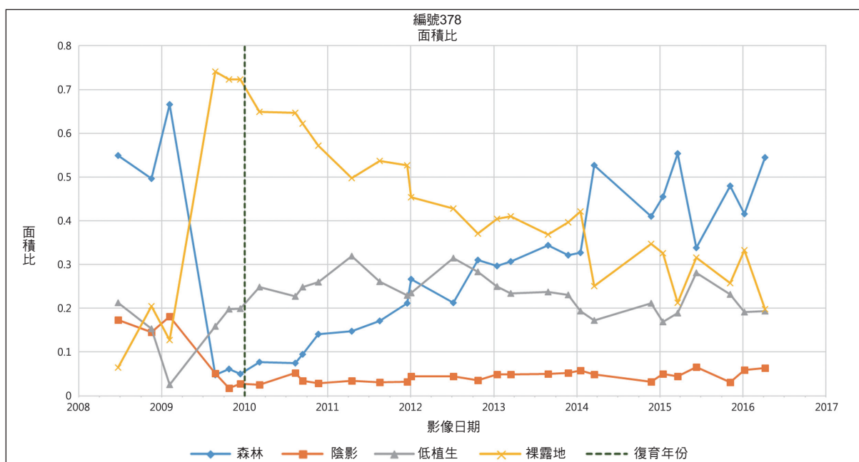
圖5、編號378樣區「森林」、「陰影」、「低植生」和「裸露地」等類型面積比例隨時間變化情形。
