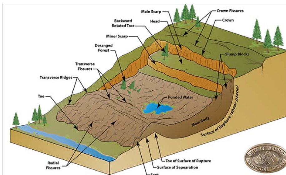
圖 2-4 弧形地滑（WSGS）
