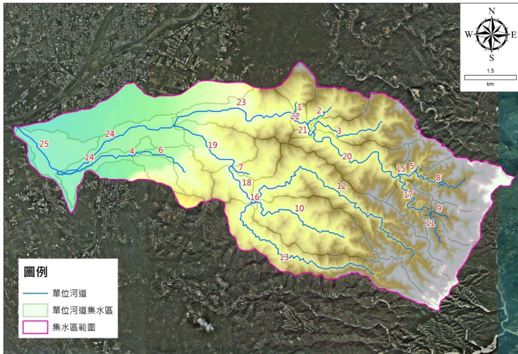
圖 4-10 草湖溪集水區單位河段編號示意圖
