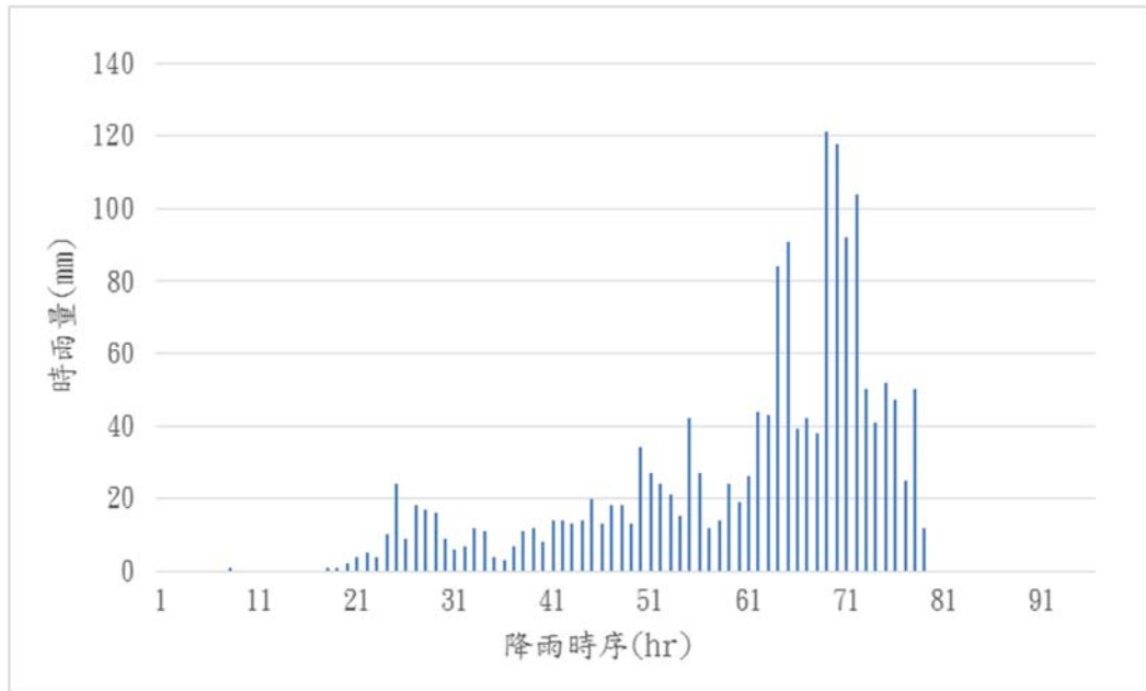
圖 4-23 莫拉克颱風(民族測站)降雨組體圖
