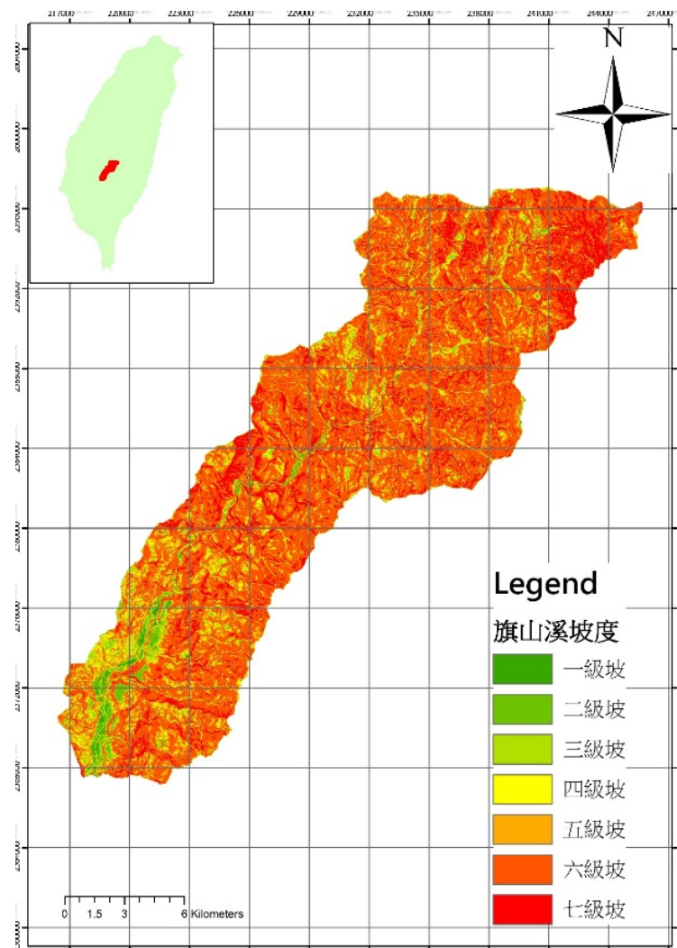
圖 4-8 旗山溪集水區坡度分布圖
