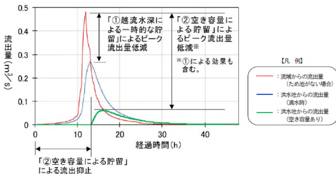
圖 5-13 農塘低水位調節示意圖 (農林水産省，2018)
