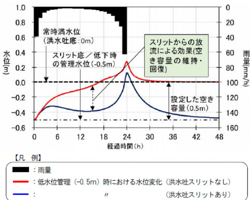
圖 5-14 溢洪道開門調節效果示意圖 (農林水産省，2018)
