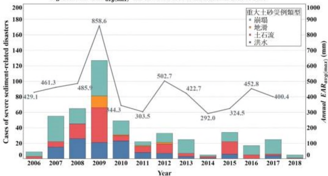
圖 6、2006-2018 年年度最大平均有效累積雨量 Annual EAR_{avg(max)} 與重大土砂災例數
