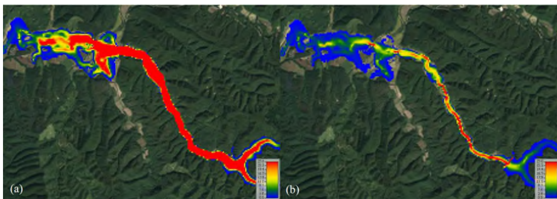
圖 4-29 潰壩水深乘流速最大分布圖: (a) Case6 (b) Case8
