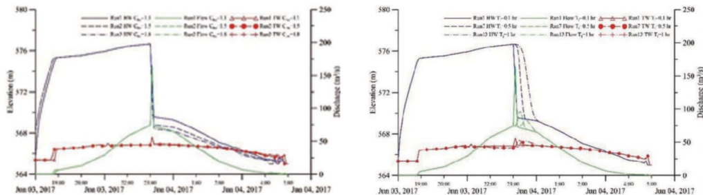
圖 9 溢流破壞水位—流量歷線圖 : (1) 潰口堰流係數變化 (Run 1, Run 2, Run 3) (左); (2) 潰壩延時變化 (Run 1, Run 7, Run 13) (右)
