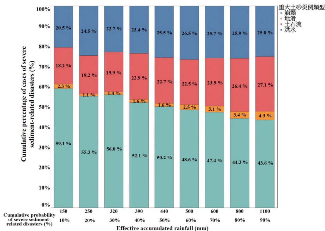
圖 4-9 不同降雨情境下之各類災害比例
