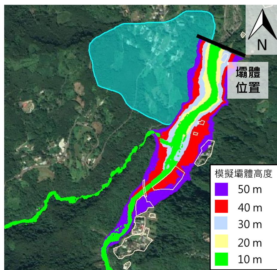
圖5.不同壩高之迴水範圍
