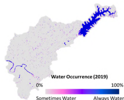
圖 2 西峨眉子集水區 地表水分布頻率圖(2019 年)
