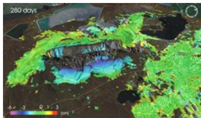
圖 2.4.1 遙測 DInSAR 進行地面變形量之分析示意圖(IRPI)
