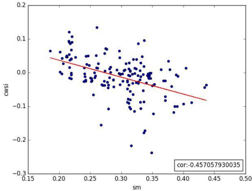
圖 3.5.10 大鳥測站 CWSI 與土壤含水量散布圖
