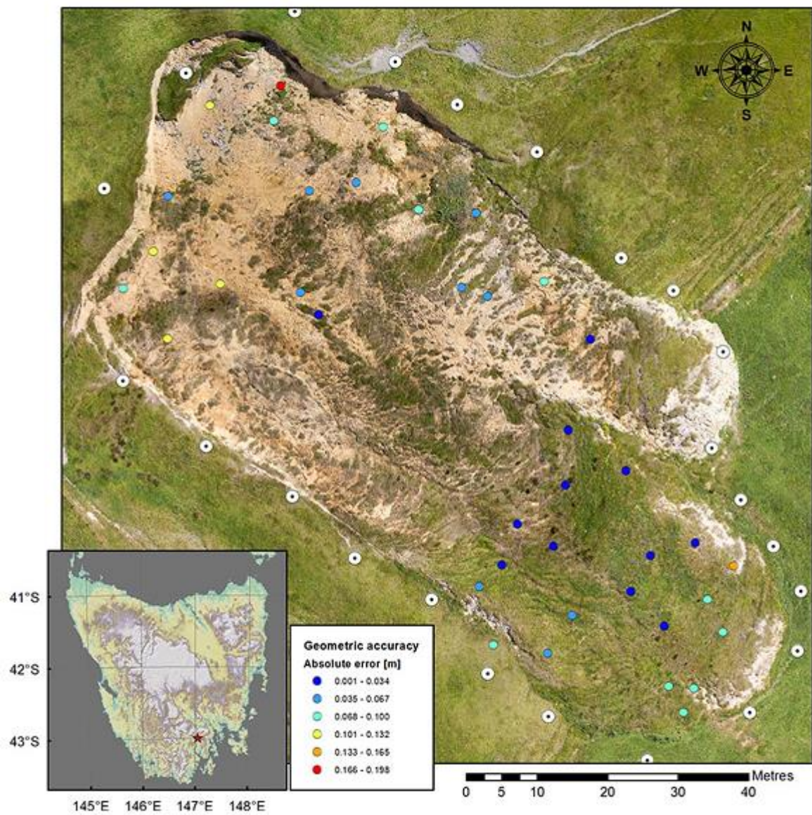
圖 3.4.7 地滑研究區監測空拍俯視圖(Lucieer et al, 2013)
