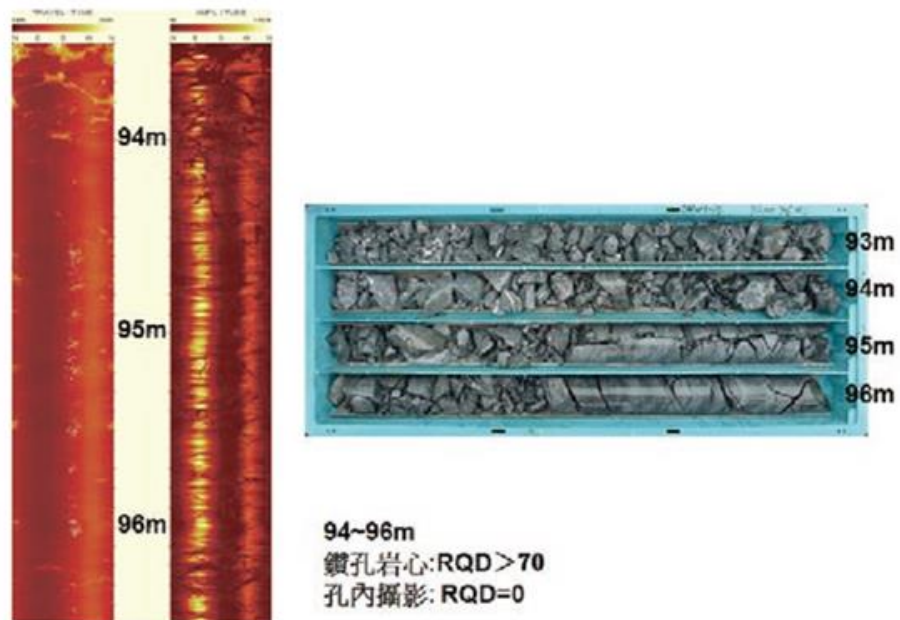
(b)鑽探與孔內攝影 RQD 之差異
