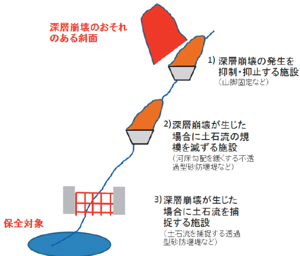
圖 3.2.22 土石流類型之硬體對策示意圖(國總研，2014)
