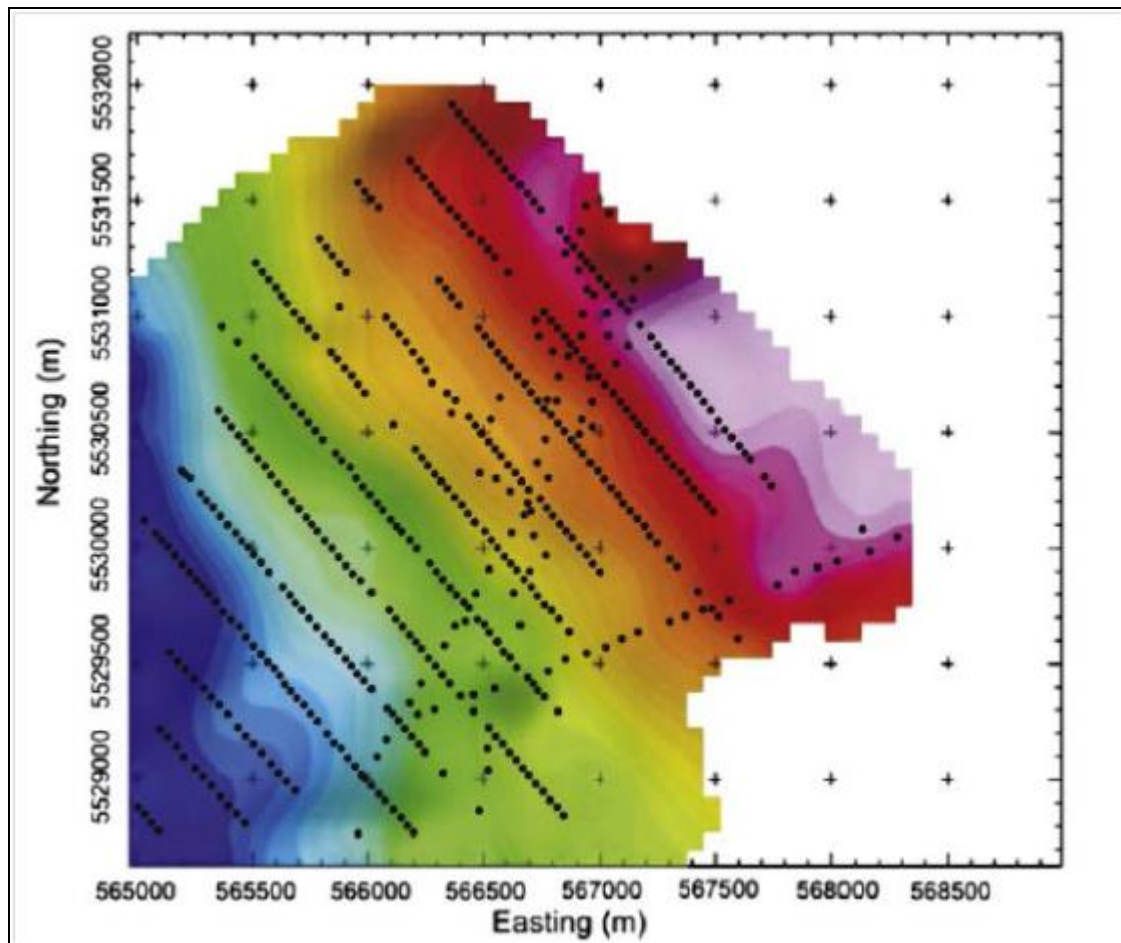
圖 3.4.15 重力探測法平面影像圖(Spicer et al., 2011)
