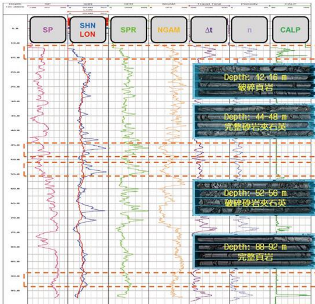
圖 3.4.21 電井測及波速調查成果示意圖(趙啟宏、羅鴻傑，2015)
