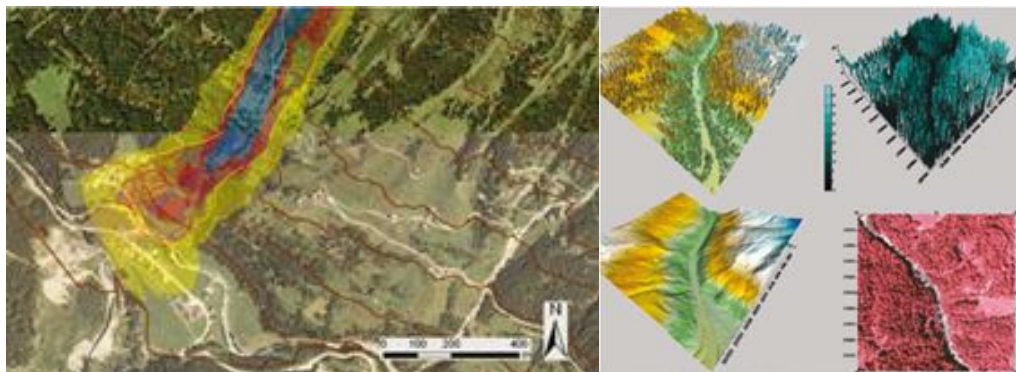
圖 2.5.2 邊坡數值模擬示意圖(防治局)
