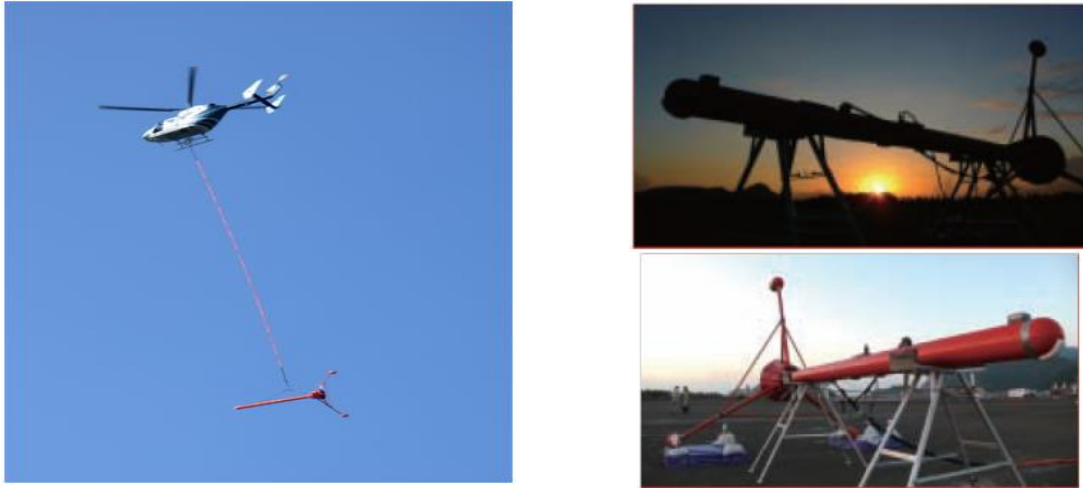
圖 3.4.9 空中磁力探測載具及感測器示意圖(工研院)
