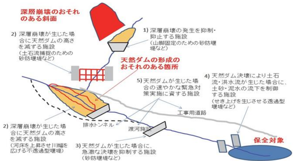
圖 4.4.3 堰塞湖類型硬體對策示意圖
