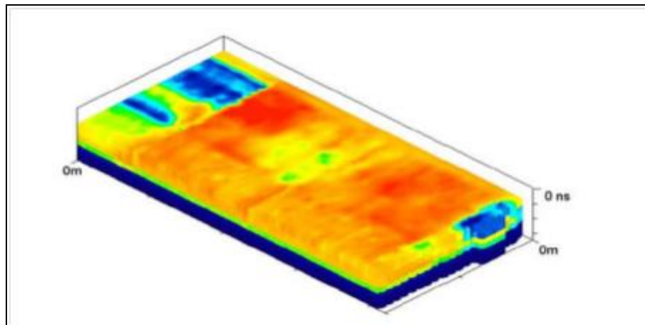
圖 3.4.13 透地雷達 3D 影像(大觀電廠溢洪道案例)
