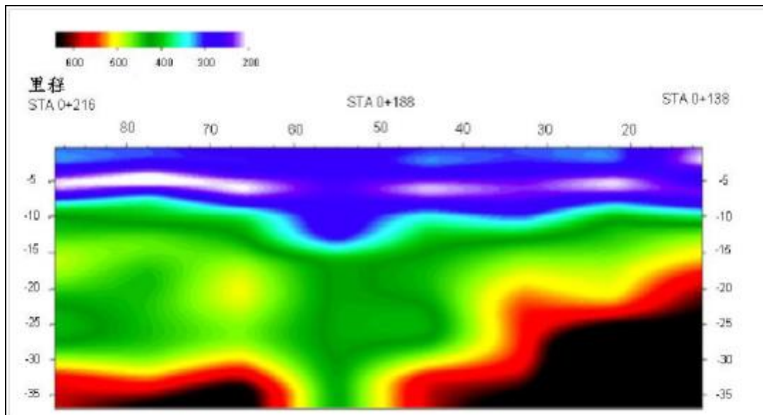
圖 3.4.17 剪力波波速影像剖面(新山水庫壩基案例)
