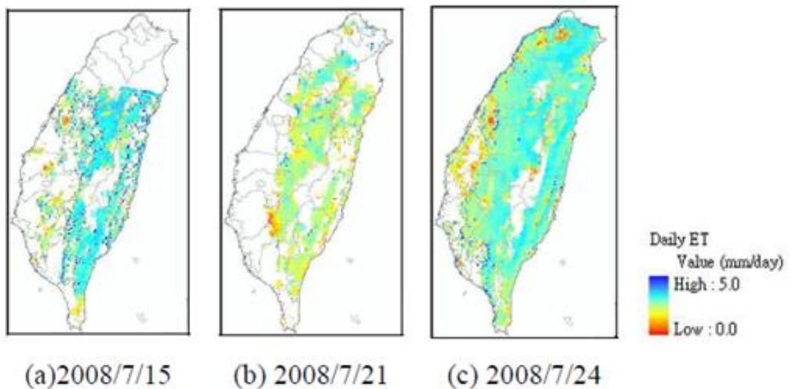
圖 4.5.5 蒸發散量示意圖(陳錕山，2009)
