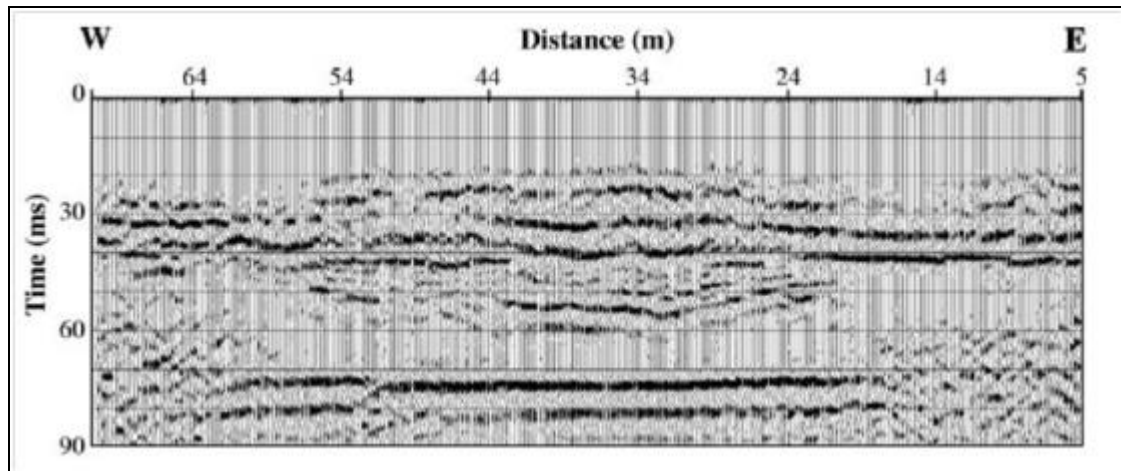
圖 3.4.18 反射震測法影像剖面(Sloan et al., 2007)
