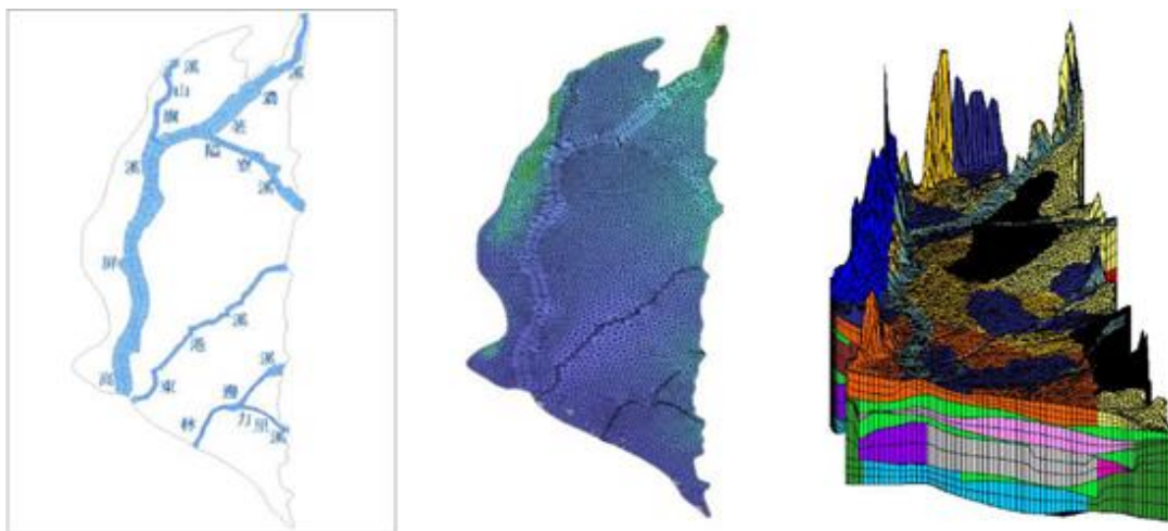
圖 2.8.4 一維河道、二維地表、三維地下模型(水利署，2015)
