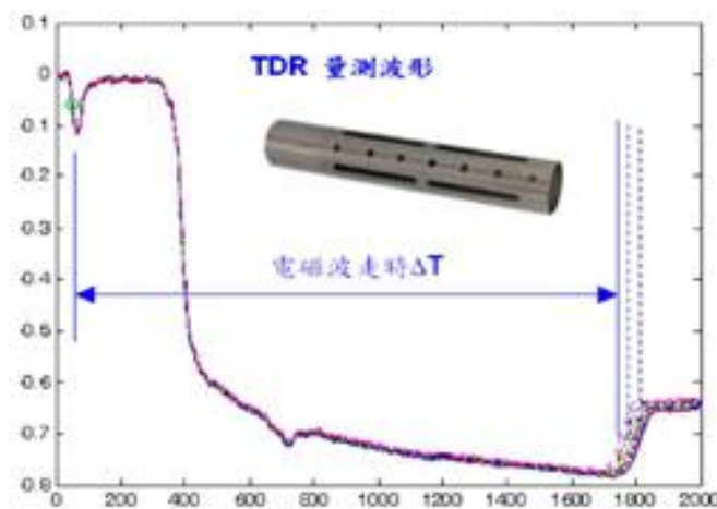
圖 2.8.2 TDR 含砂濃度感測器與量測典型波形(水利署，2015)
