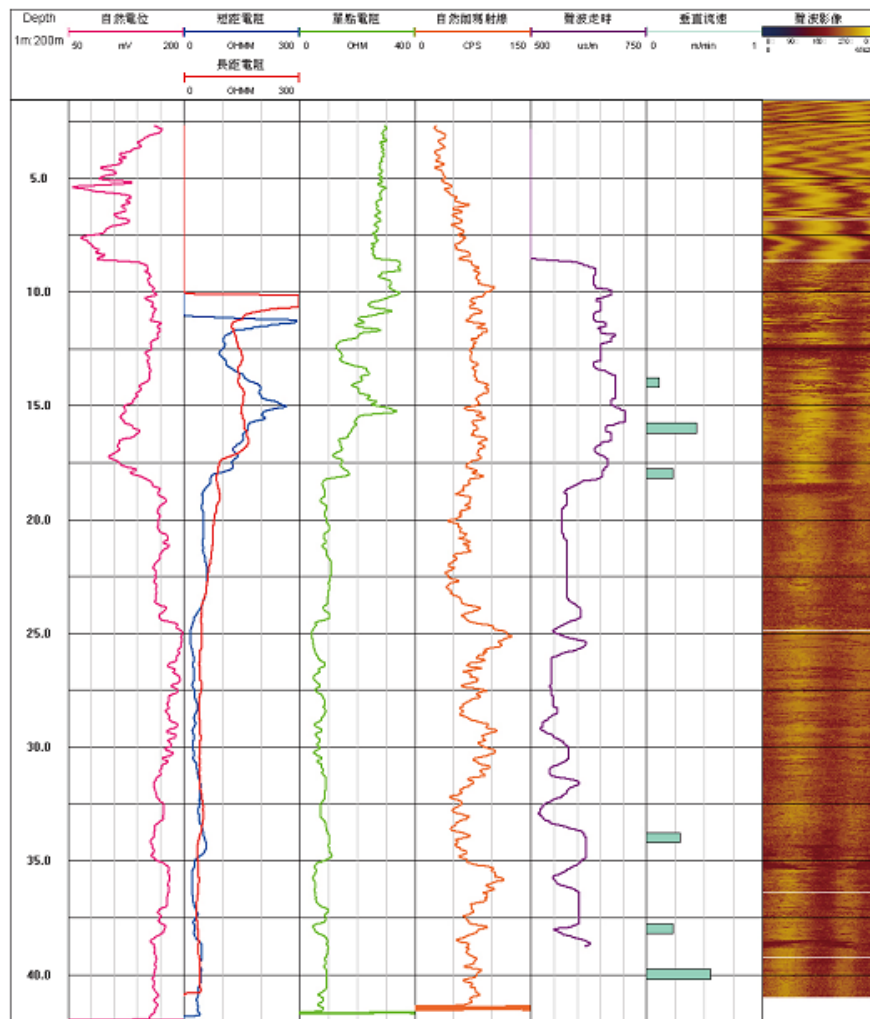
圖 3.4.23 孔內探測調查結果示意圖(趙啟宏、羅鴻傑，2015)
