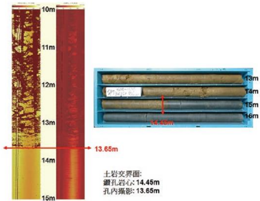
(a)鑽探與孔內攝影深度錯位情形
