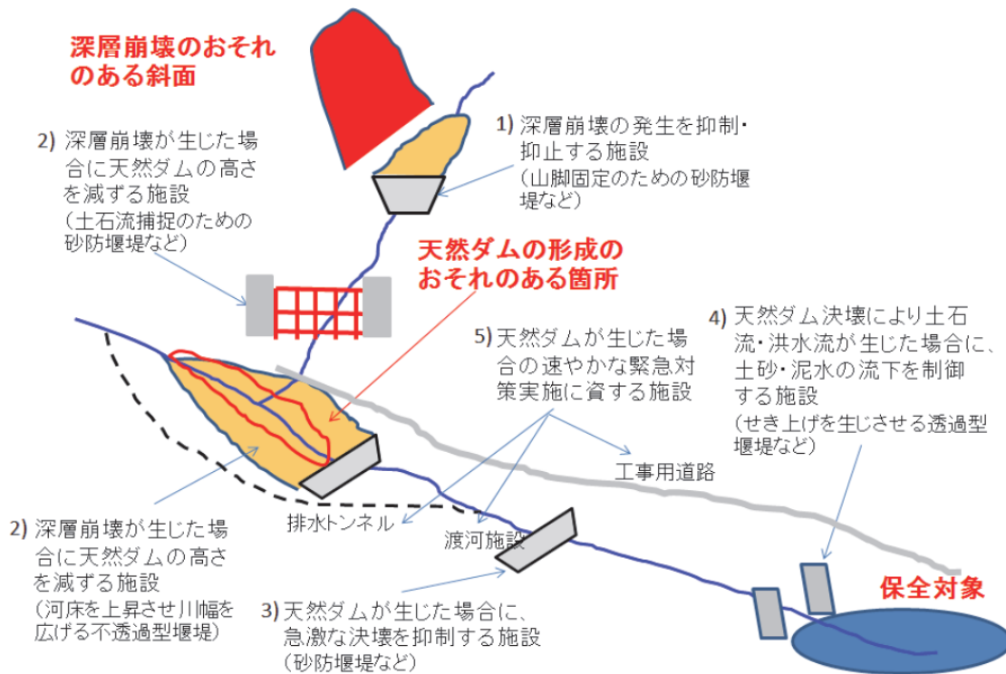
圖 3.2.21 堰塞湖類型之硬體對策示意圖(國總研，2014)
