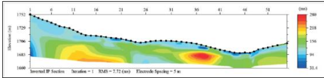
圖 3.4.12 感應極化法影像剖面圖(Advanced Geosciences Inc., 2010)
