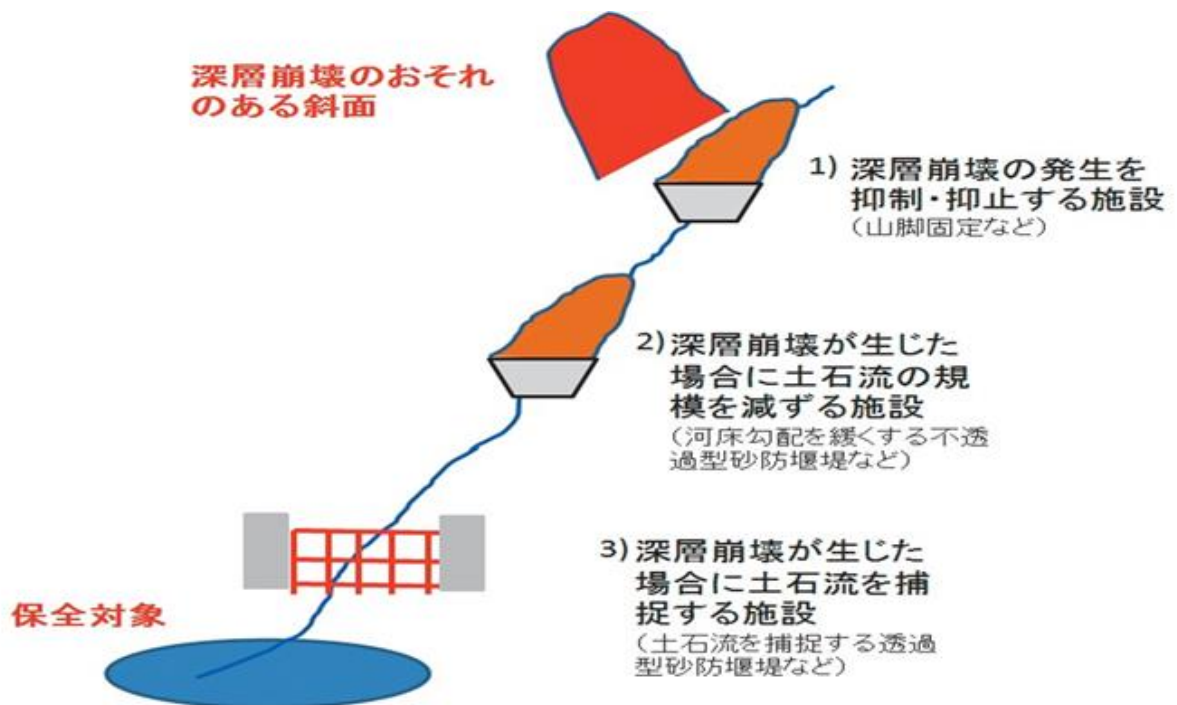
圖 4.4.4 土石流類型硬體對策示意圖
