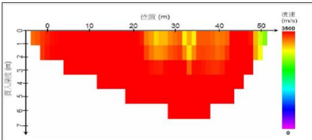
圖 3.4.16 壓縮波波速影像剖面圖(石門水庫廊道案例)
