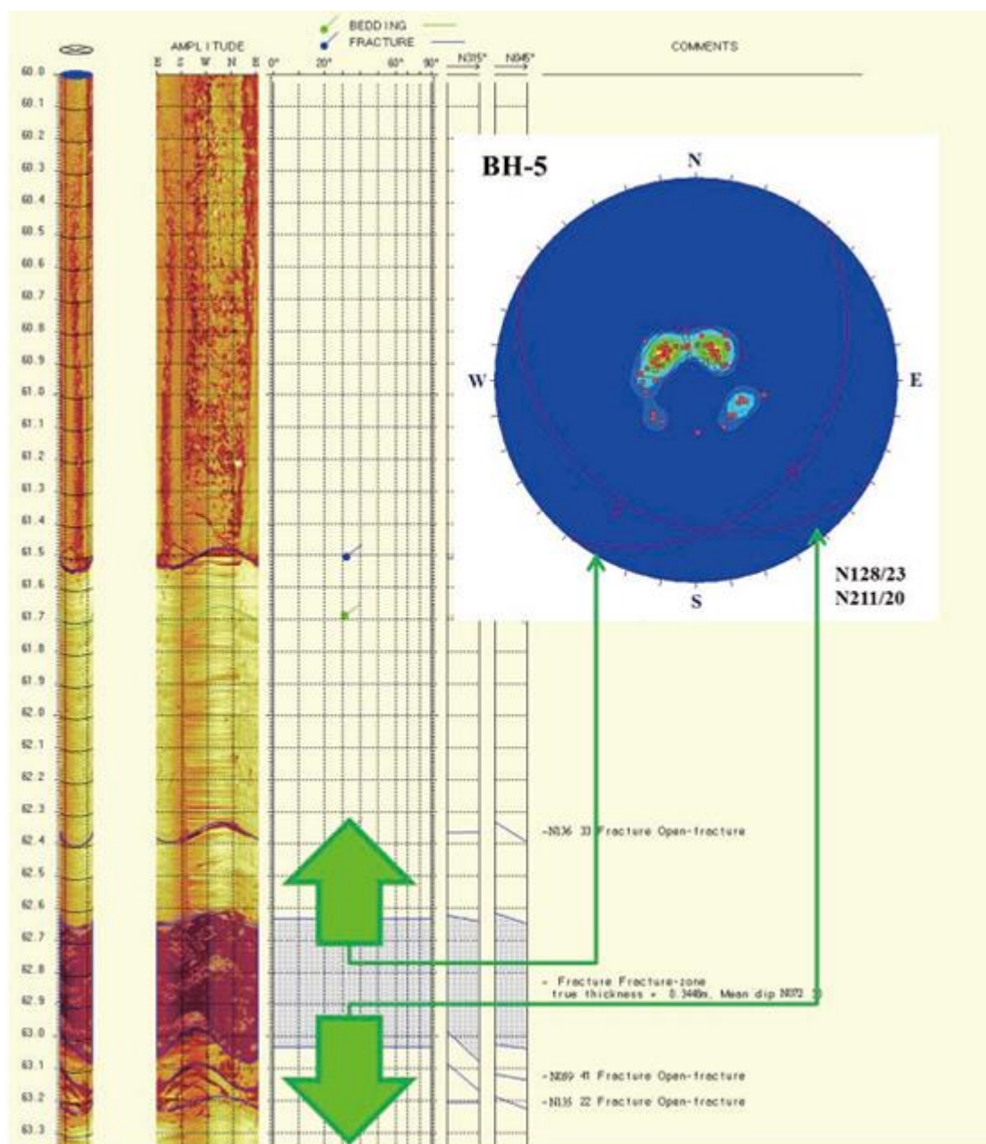
圖 3.4.20 鑽孔內不連續面位態隨深度變化情形示意圖
