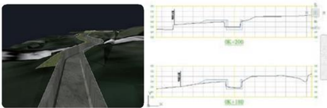
圖 3.1.1 地形、設計縱坡及組合斷面產生 3D 廊道及溝渠橫斷面示意
