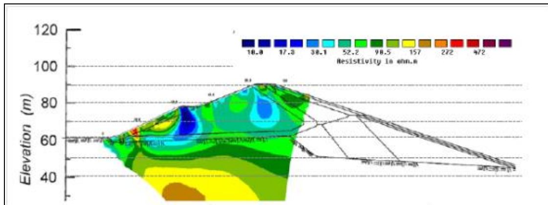
圖 3.4.10 電阻率影像剖面圖 (新山水庫案例)
