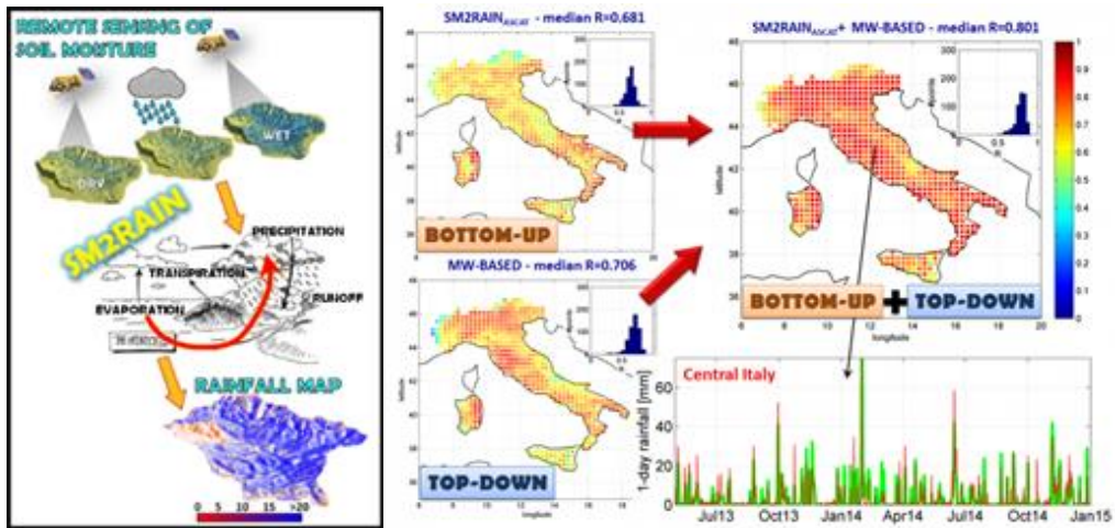
圖 2.4.2 遙測衛星估算土壤含水量並建立降雨量估算系統 (SM2RAIN) (IRPI)
