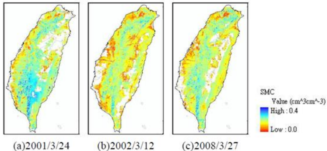
圖 4.5.6 土壤含水量分析示意圖(陳錕山，2009)
