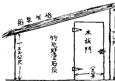
圖二：家庭雞舍側面
