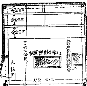
圖四：家庭雞舍平面
