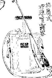
圓桶型 理想噴霧器
