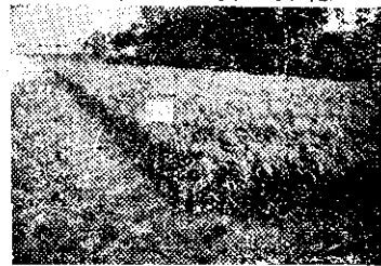
在彰化縣農林改良場經處理「土蘭師扶朗多旺」茂盛生長的稻田
