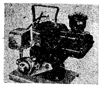
美國某公司最近創製一種手提式抽水機，構造簡單，輕巧實用。這種抽水機，可用做噴霧及灌溉園地之用。當抽水工作完畢後，它會自動關閉，所以使用時不必費力。抽水機，每臺重僅卅五磅，一分鐘可以抽水八加侖，壓力卅呎，噴水高度可達卅英尺。
