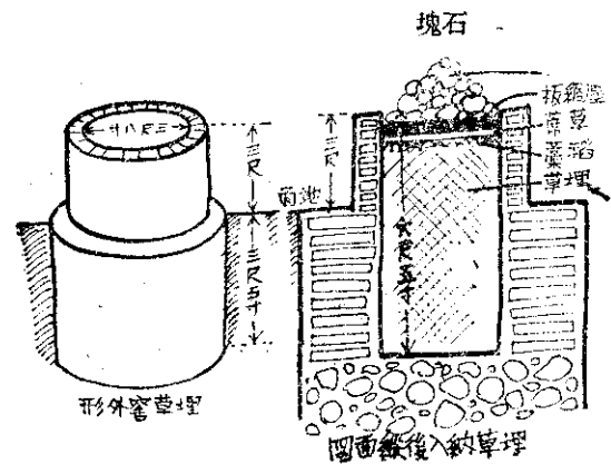
農家小用埋草窖設計圖
