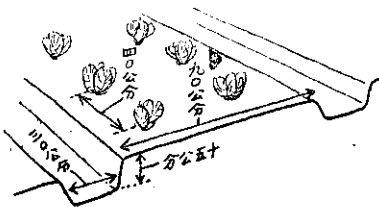
本圃畦高五十公分，分五公分，畦寬九十分，分三公分，每行栽二株，行距四十分，每畧十公畝地種四千株。
