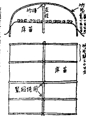
玻璃布苗床的正面圖（上）與平面圖
