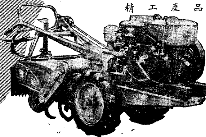
H18 型耕犁機
