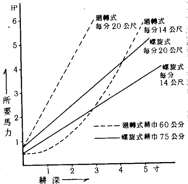
日本九州大學農學部調查結果 同一耕速下迴轉式與螺旋式之特性比較
