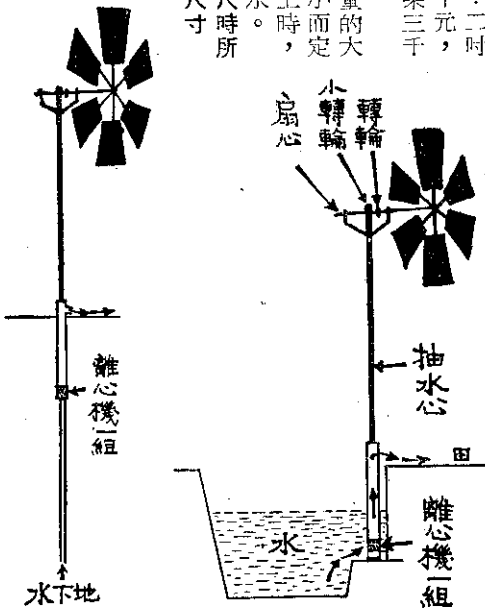
風力抽水機圖解
