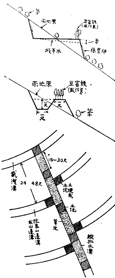
圖三：蓄水土堤和土坑的佈置
