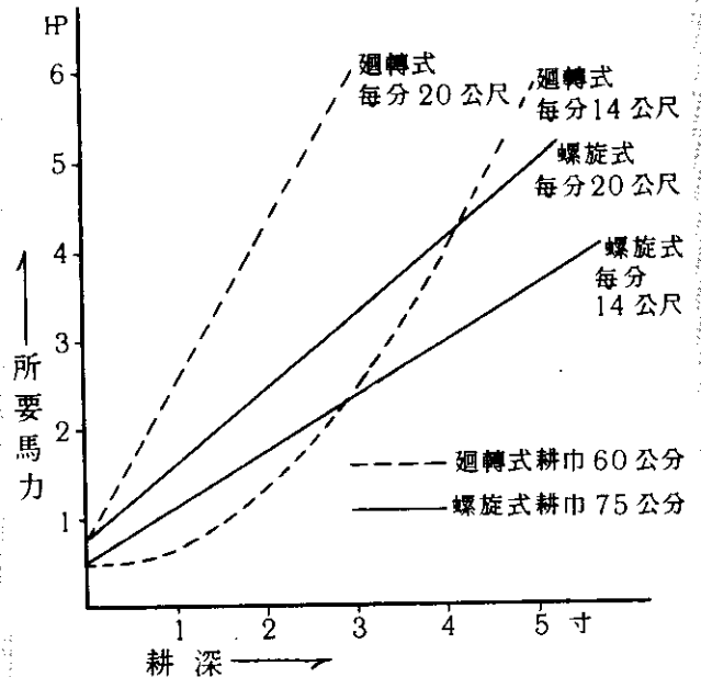
日本九州大學農學部調查結果 同一耕速下迴轉式與螺旋式之特性比較
