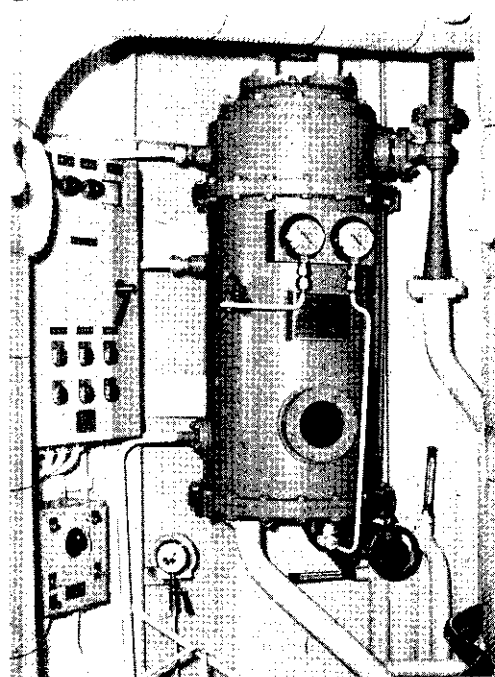
海水變淡水的裝置。
